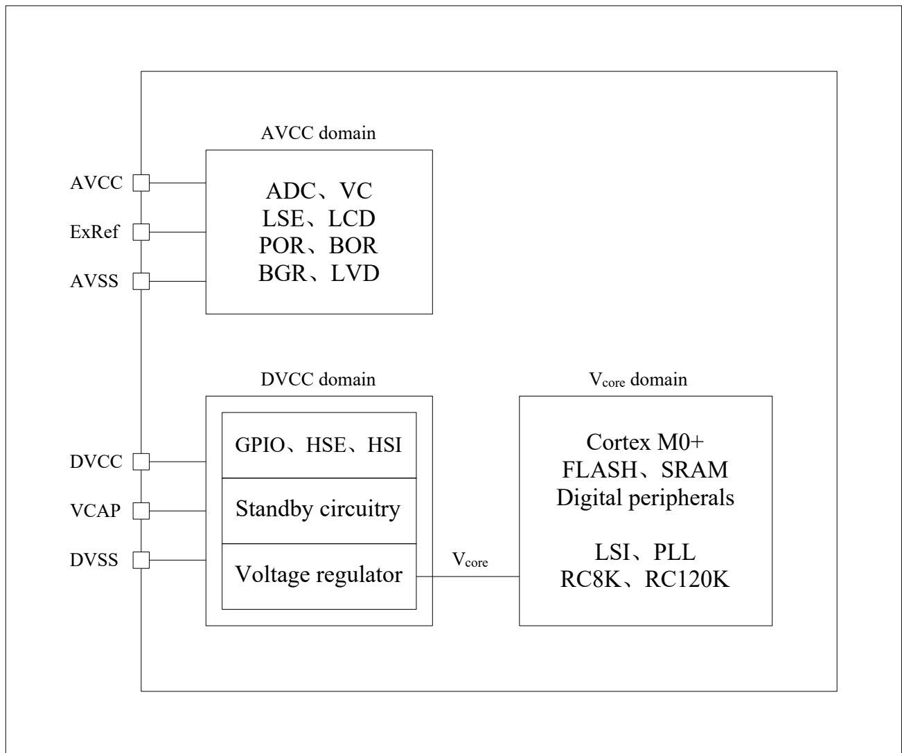
图 8-3 电源系统
