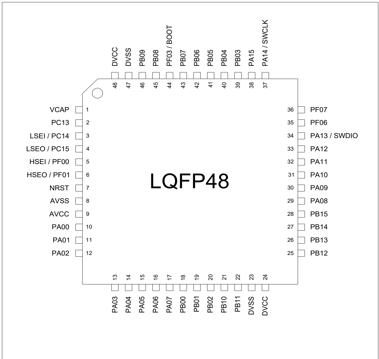
图 4-4 LQFP48 管脚定义
