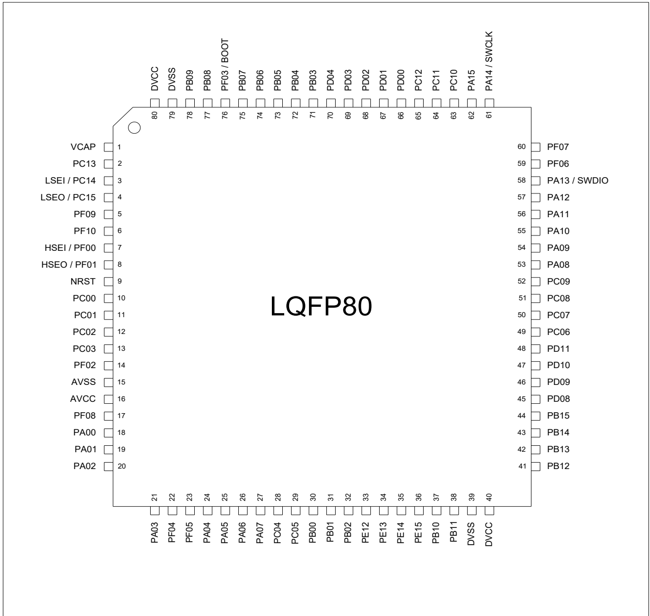
图 4-2 LQFP80 管脚定义
