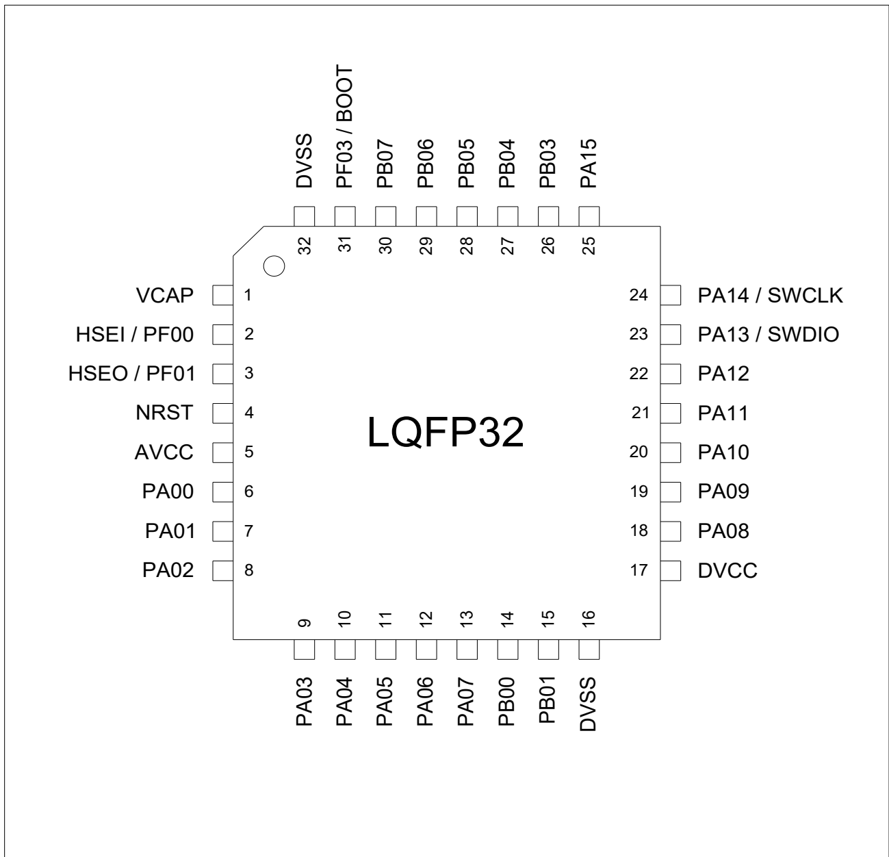
图 4-6 LQFP32 管脚定义
