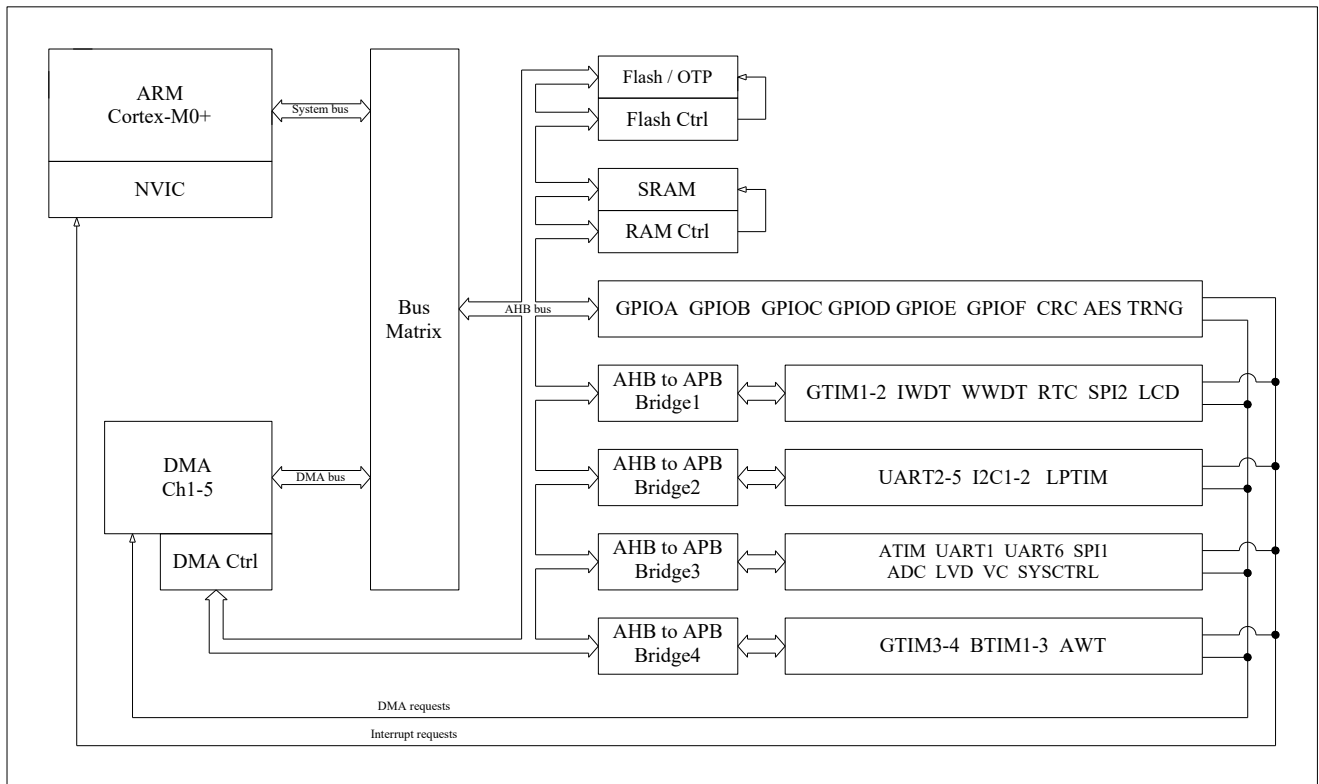
图 5-1 功能框图
