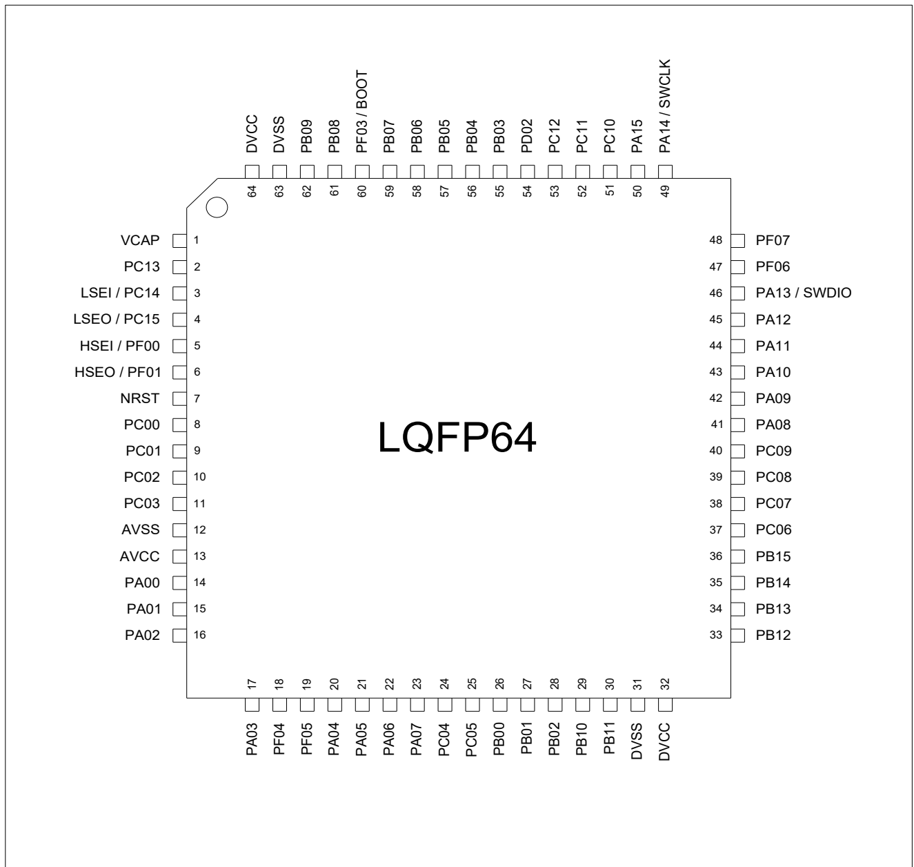
图 4-3 LQFP64 管脚定义
