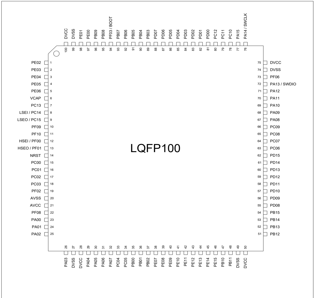
图 4-1 LQFP100 管脚定义
