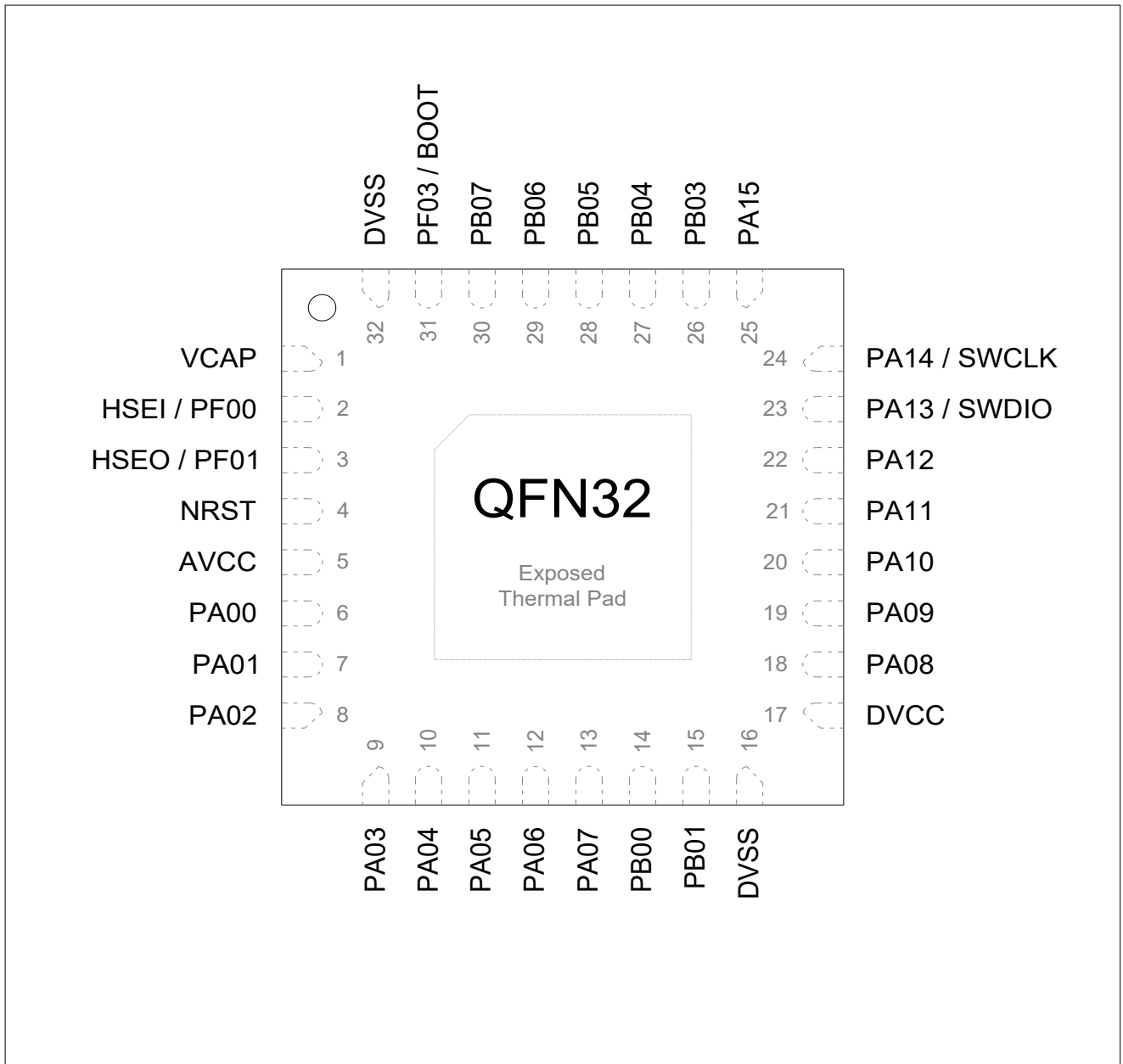
图 4-7 QFN32 管脚定义
