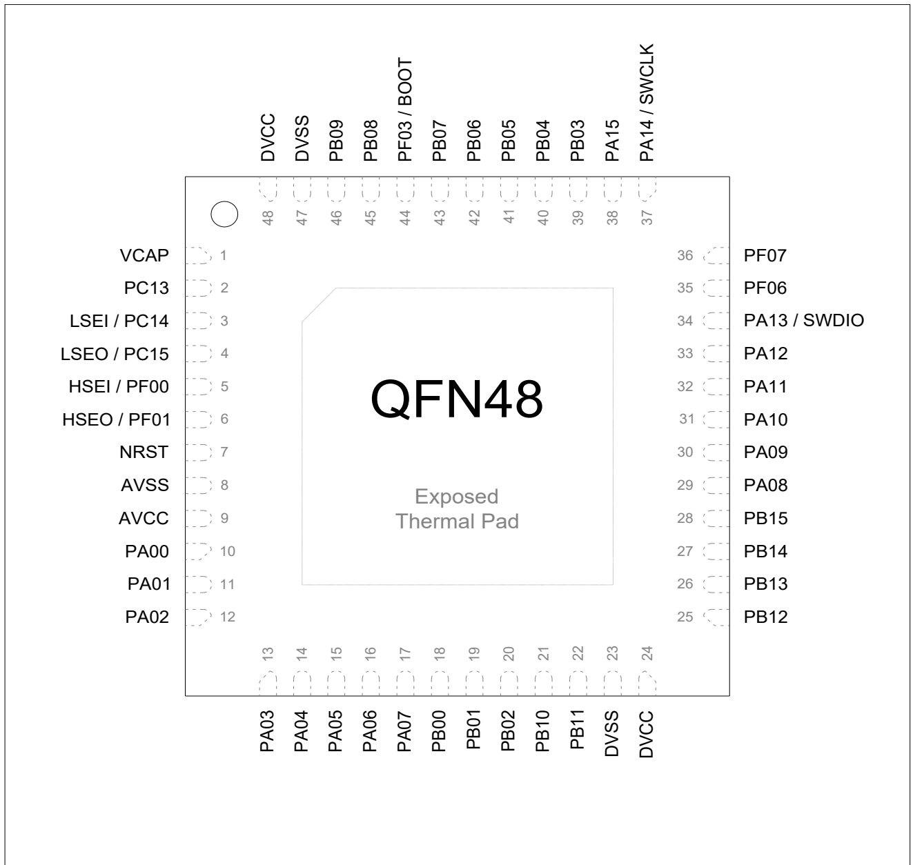
图 4-5 QFN48 管脚定义
