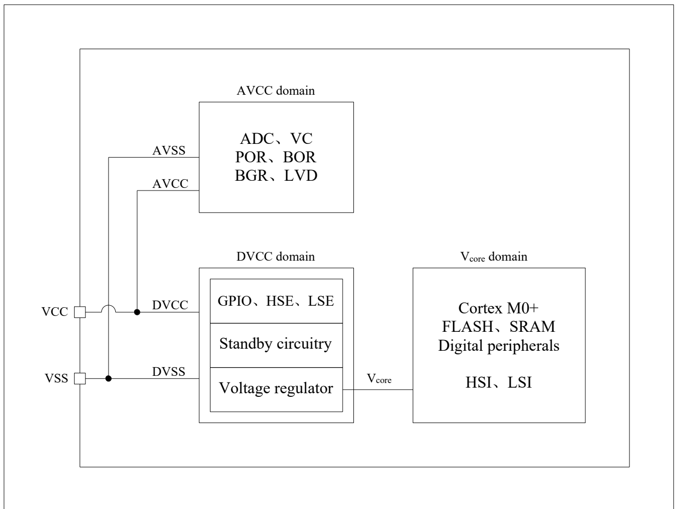
图 8-3 电源系统
