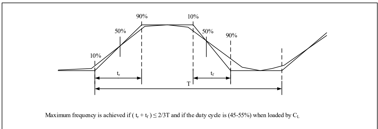
图 8-8 I/O 口交流特性定义
