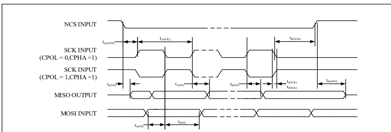
图 8-12 SPI 时序图 – 从机模式 CPHA=1
