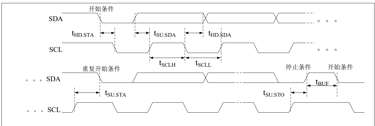
图 8-10 I2C 时序图
