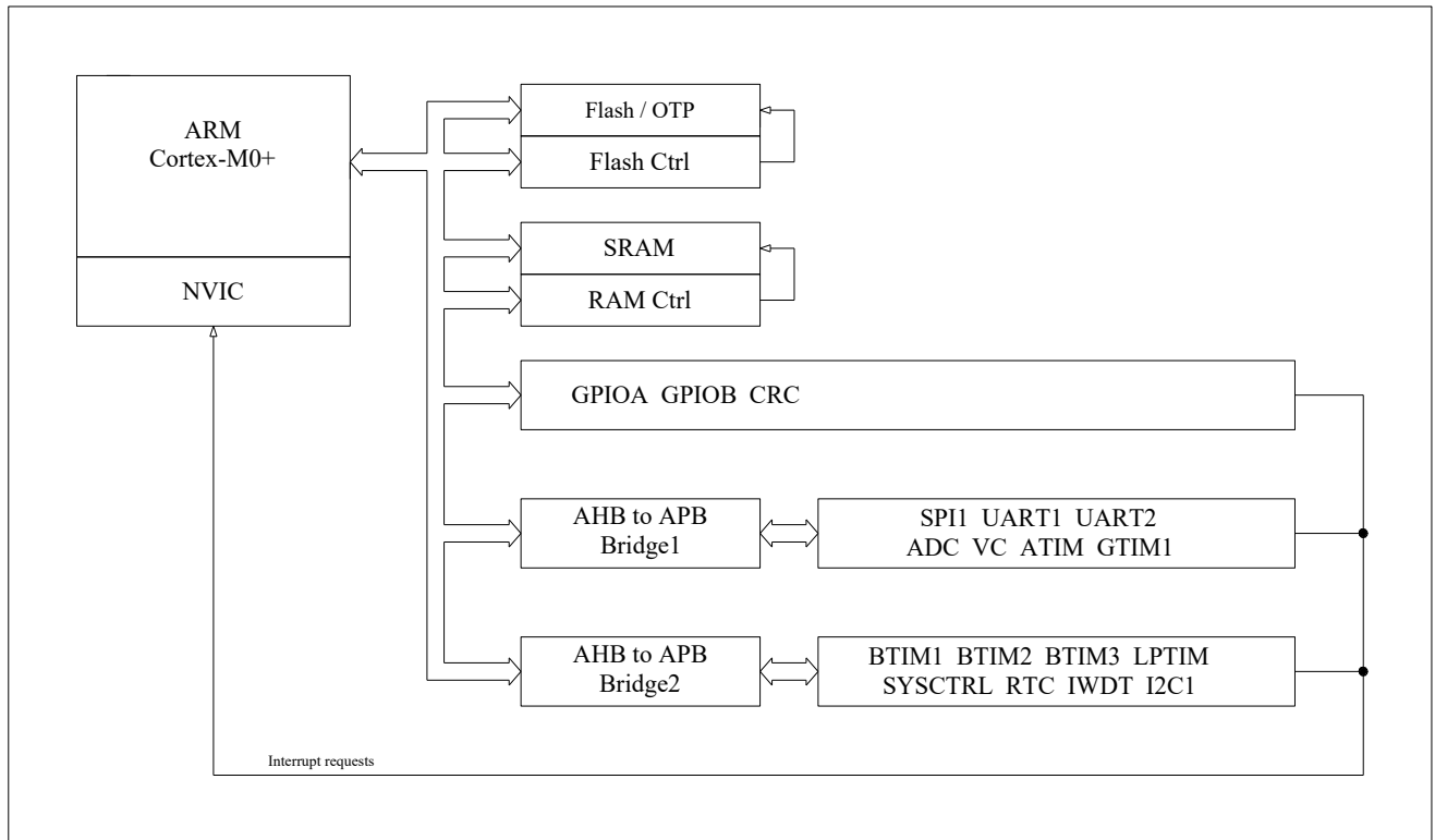
图 5-1 功能框图
